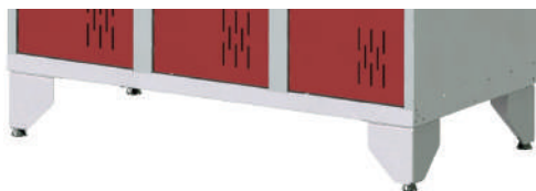
Pés elevatórios em aço galvanizado código 22.60.00.01
