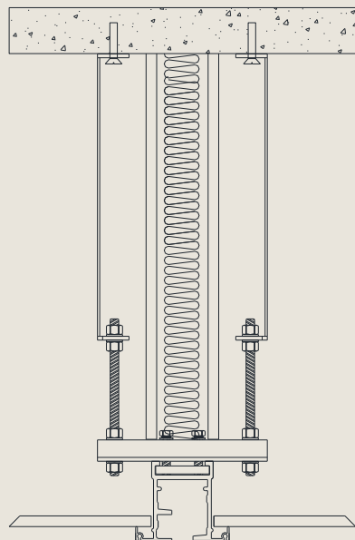
Fixação sob Laje através de chumbadores
