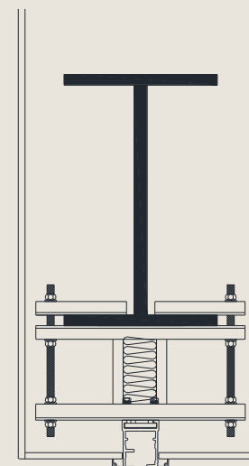
Fixação sob viga "I" através do sistema de castanhas
