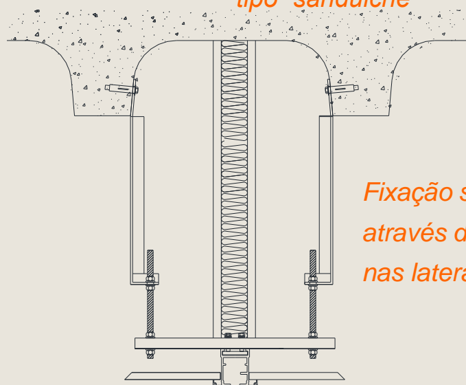
Fixação sob treliça metálica através do sistema tipo "sanduiche"
