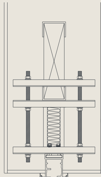
Fixação sob treliça metálica através do sistema tipo "sanduiche"
