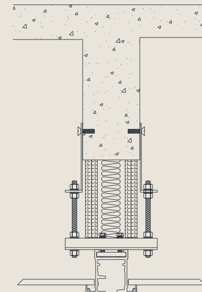
Fixação sob viga de concreto através de chumbadores nas laterais da viga
